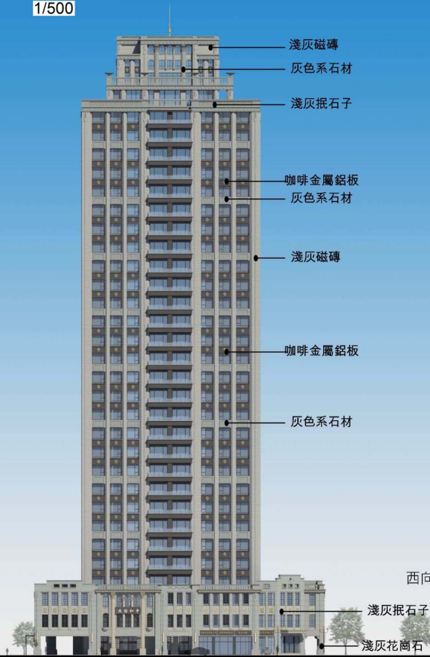
北向立面圖
